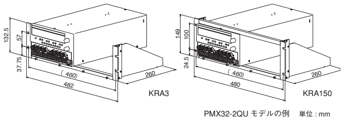
PMX32-2QU モデルの例 単位: mm
