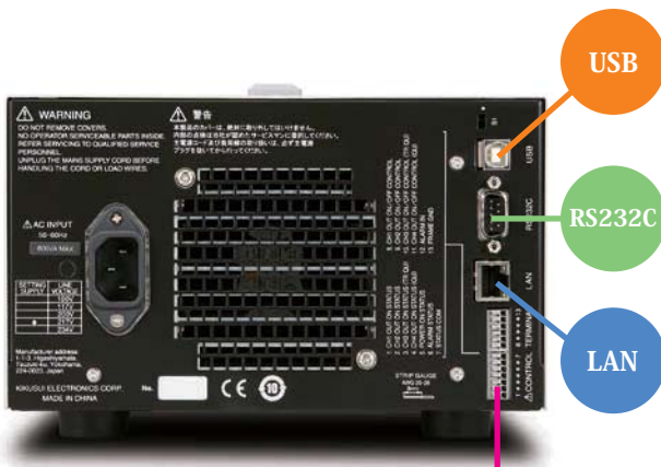
外部コントロール用端子台
